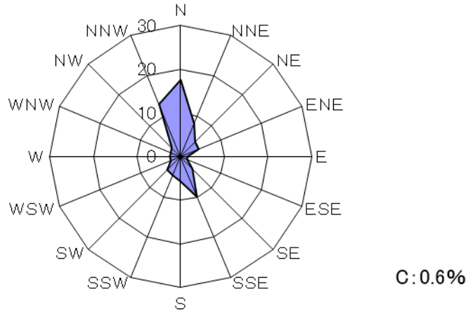
年間風配図
