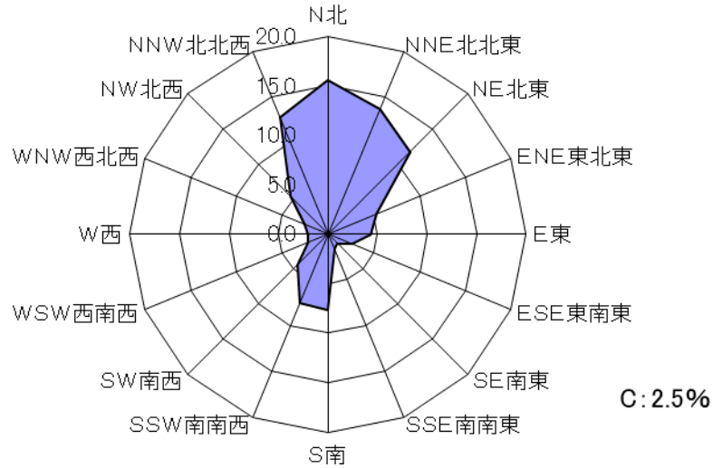
年間風配図
