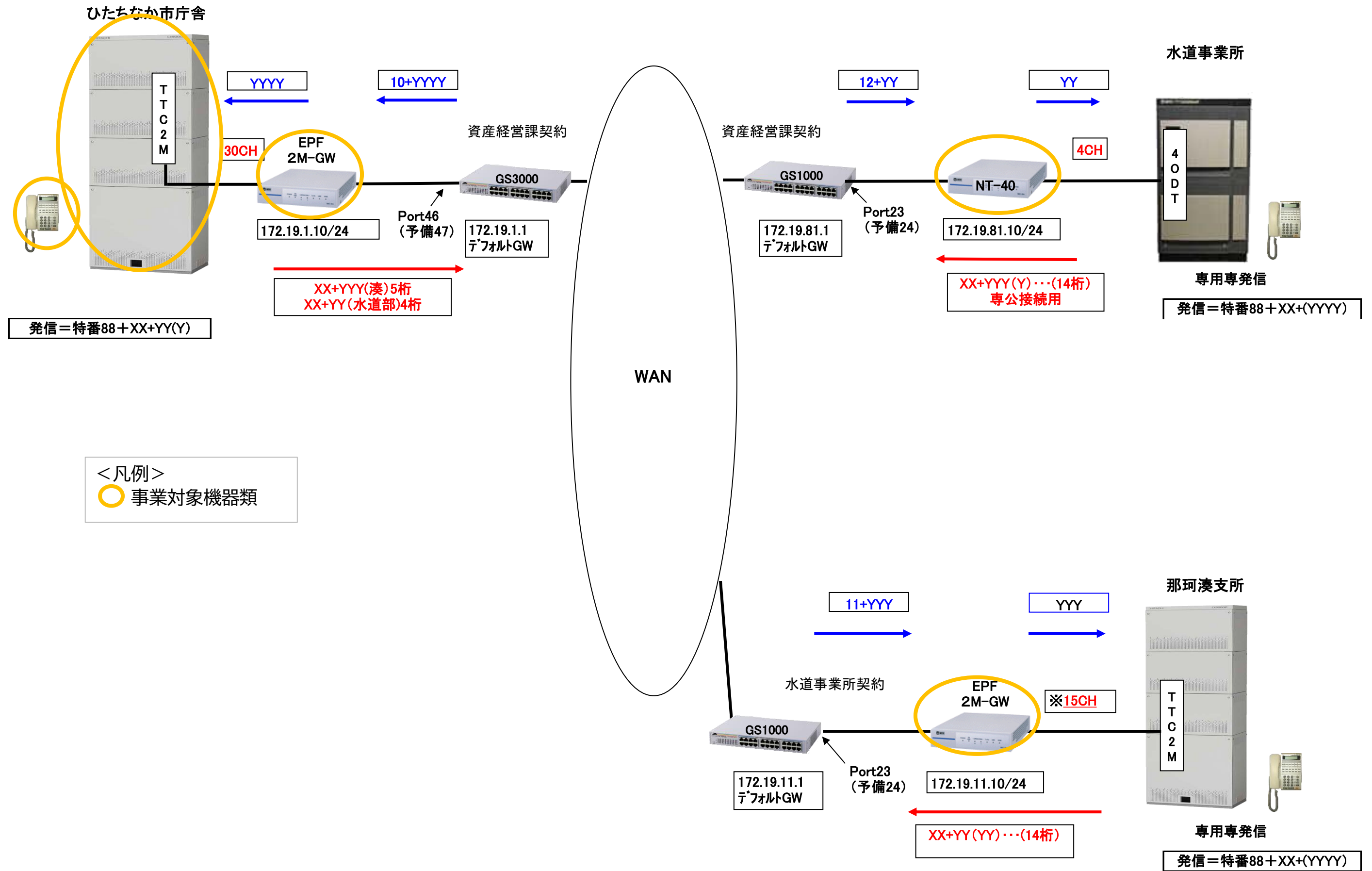
IP専用線ネットワーク構成図
