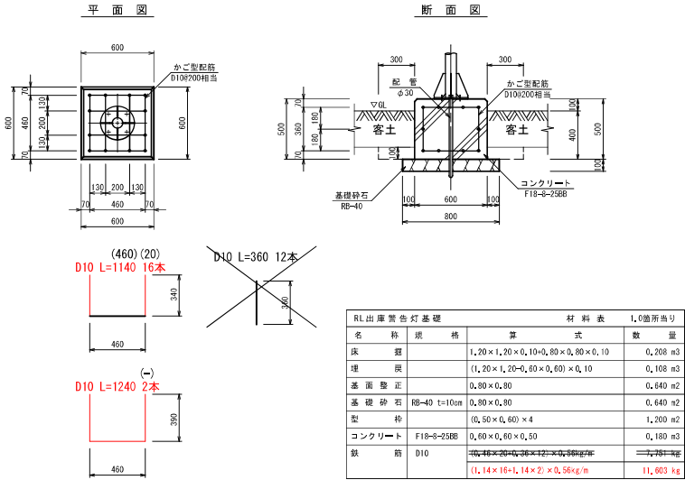
RL出庫警告灯基礎 S=1:20
