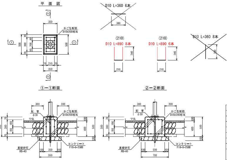
BCバーキャッチャー基礎 S=1:20
