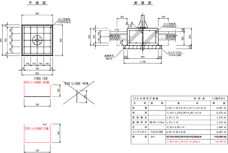
ES入口表示灯基礎 S=1:20
