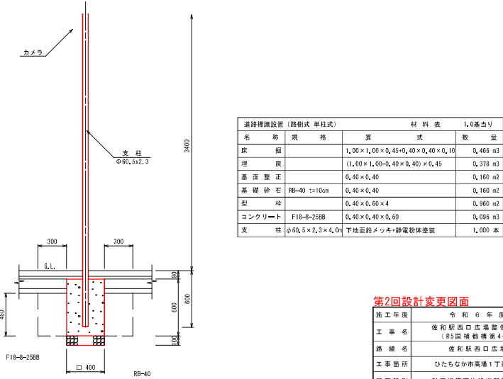
カメラポール設置標準図 S=1:20
