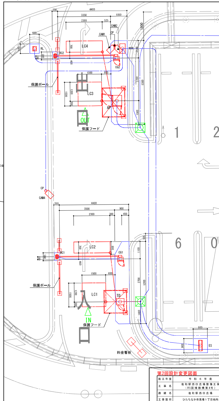
出入口拡大図 Sc.1/50 (A1)
