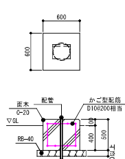
RL基礎 詳細図 SC.1/30(A1), 1/60(A3)
