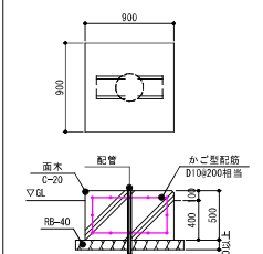
ES基礎 詳細図 SC.1/30(A1), 1/60(A3)
