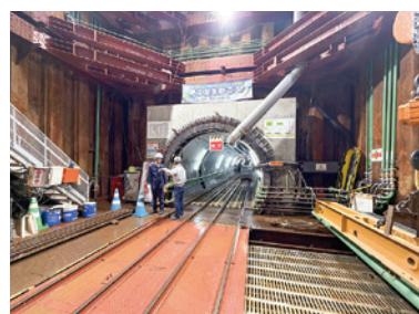
大島第2幹線管きょ布設工事の様子
