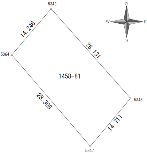
< 地積測量図 >
